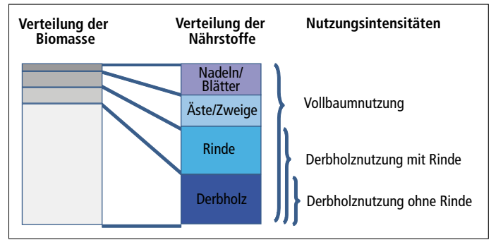
Abb. 2: Schema der Biomasse und Nährstoffentzüge durch unterschiedlich intensive Nutzung
