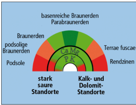
Abb. 1: Nährstoffverfügbarkeit in Abhängigkeit der Bodenreaktion
